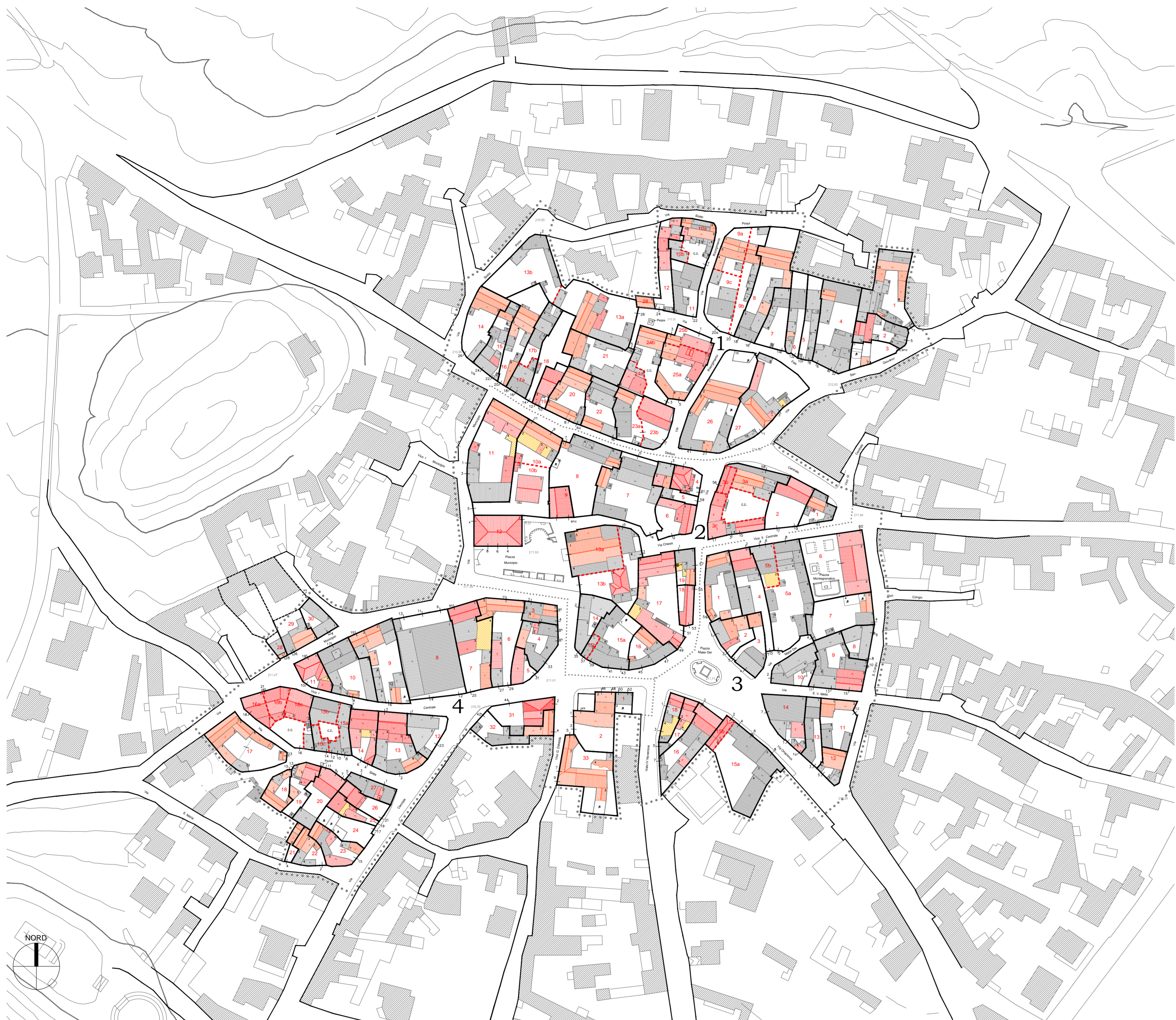
GEOMETRIA DELLE COPERTURE DI STATO ATTUALE scala 1:1000
